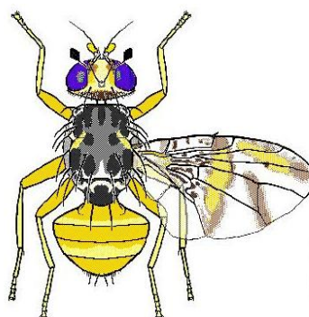
Ceratitidis capitata
